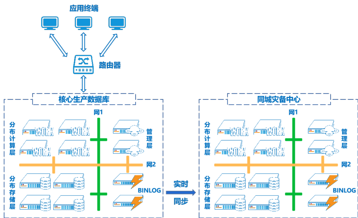
图 1-2 同城灾备
