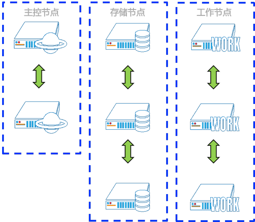
图 1-9 存算分离
